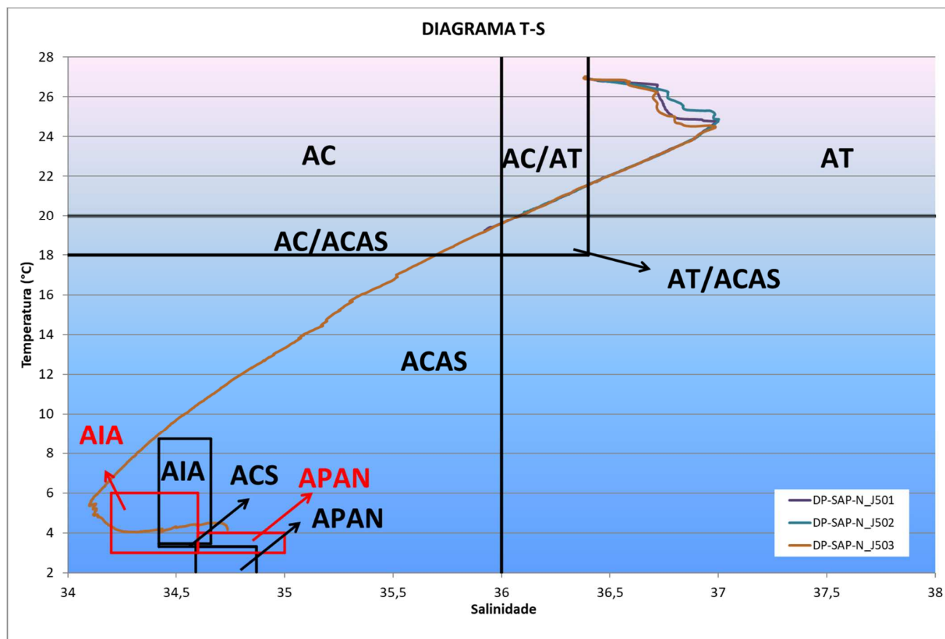
Figura V-5 – Diagrama T-S do DP-SAP-N_C6. Em preto, limites estabelecidos por Tommasi (1994) e Silveira et al. (2000) e em vermelho, limites estabelecidos por Castro et al. (2006).
