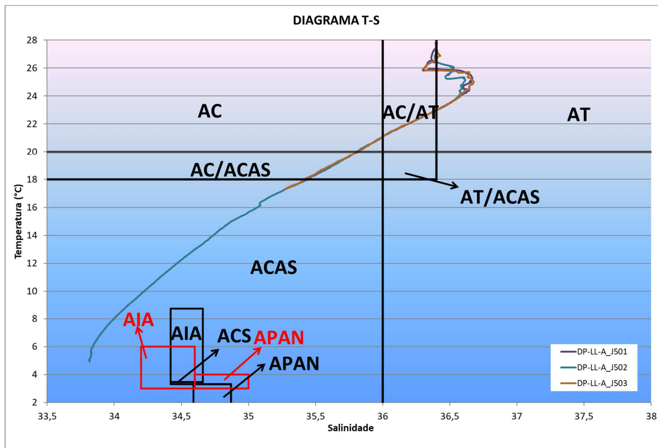
Figura V-3 – Diagrama T-S do DP-LL-A_C4. Em preto, limites estabelecidos por Tommasi (1994) e Silveira et al. (2000) e em vermelho, limites estabelecidos por Castro et al. (2006).
