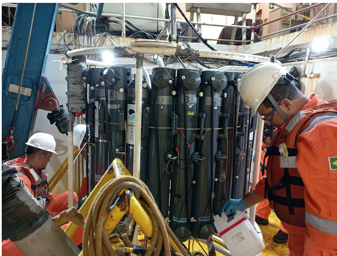
Figura IV-4 – Rosette com garrafas de coleta de amostras de água dos modelos Niskin e Go-flo utilizadas no atual ciclo de monitoramento.
