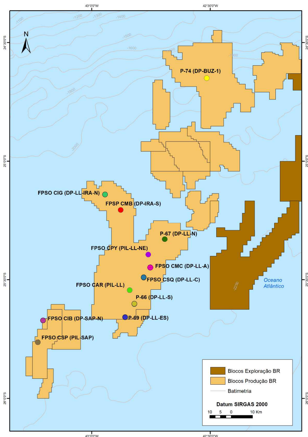
Figura IV-5 – Áreas de produção com a localização dos FPSOs do PM500: FPSO CIB (DP-SAP-N), FPSO CSQ (DP-LL-C), FPSO CIG (DP-LL-IRA-N), FPSO CMC (DP-LL-A), P-66 (DP-LL-S) e P-69 (DP-LL-ES) e das unidades usadas como referências para comparação dos resultados: FPSO CSP (PIL-SAP), FPSO CAR (PIL-LL), FPSO CMB (DP-IRA-S), P-74 (DP-BUZ-1) e FPSO CPY (PIL-LL-NE).
