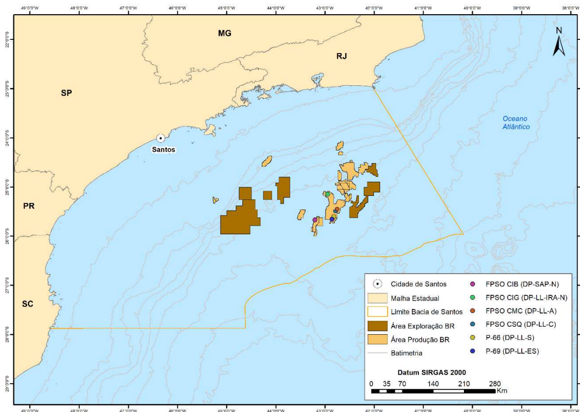
Figura III-1 - Localização das unidades amostradas durante o PM500-BS_C6: FPO CIB (DP-SAP-N), FPO CSQ (DP-LL-C), FPO CIG (DP-LL-IRA-N), P-66 (DP-LL-S), FPO CMC (DP-LL-A) e P-69 (DP-LL-ES) sobrepostas às áreas de Exploração e Produção da Petrobras da Bacia de Santos.
